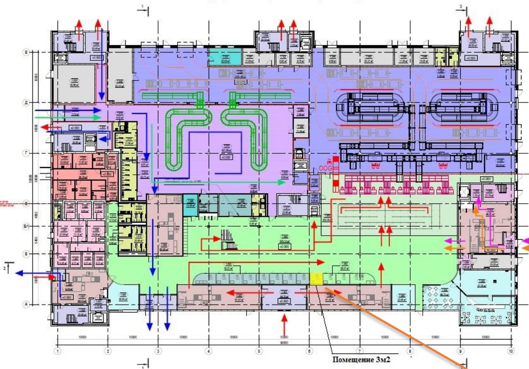
План функционального зонирования 1-го этажа (на отм. 0.000)
