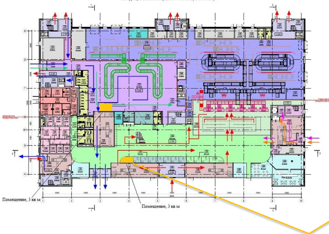
План функционального зонирования 1-го этажа (на отм. 0.000)
