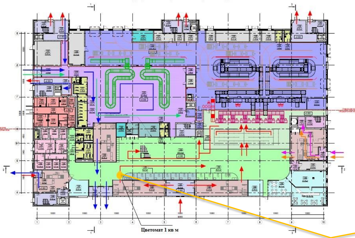
План функционального зонирования 1-го этажа (на отм. 0.000)
